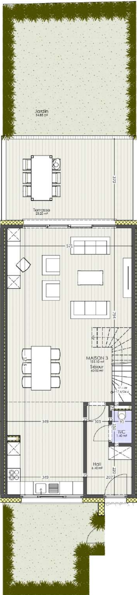
REZ-DE-CHAUSSEE
